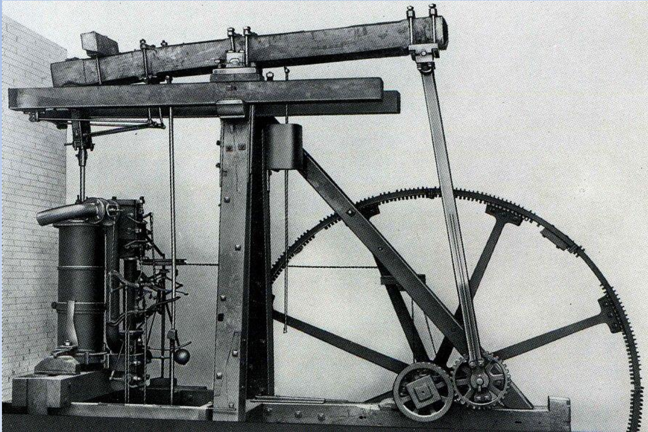
Dampfmaschine von James Watt (1773)
