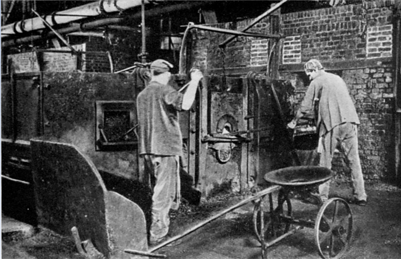
Puddelofen. Puddelverfahren von Henry Court (1784) ersetzt Holzkohle durch Steinkohle als Brennstoff
