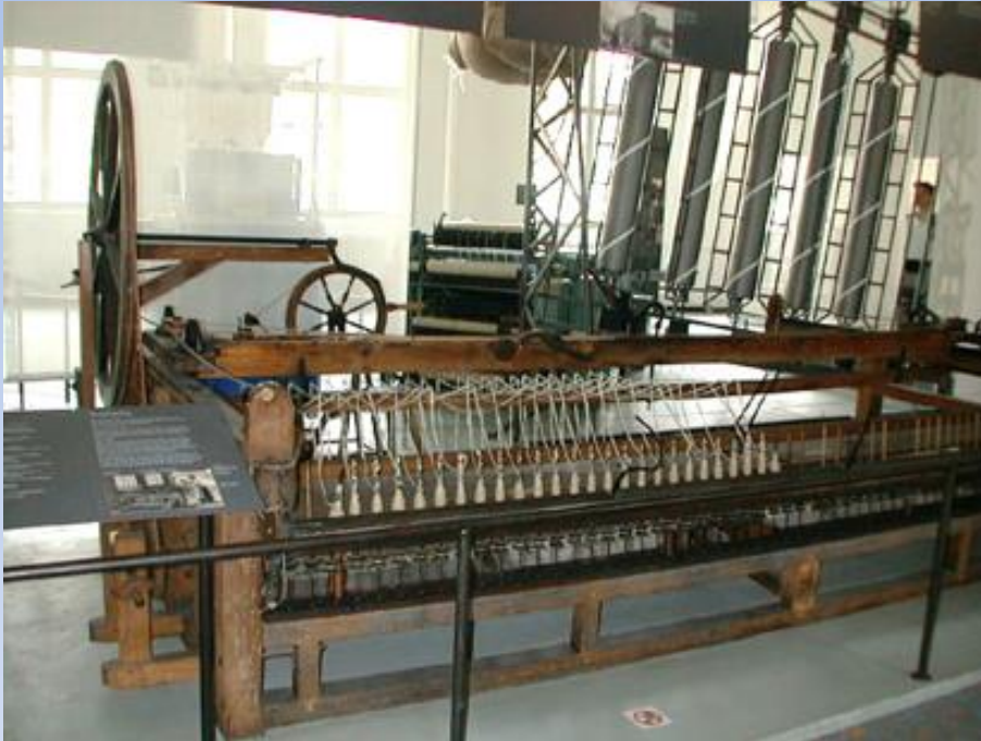
James Hargraves „Jenny“ (1767)
